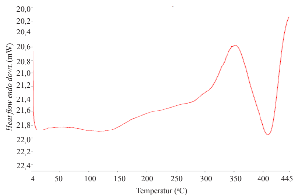
Gambar 10. DSC vulkanisat karet alam/butil (65/35) phr sistem CV.
