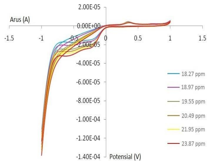
Gambar 3. Cyclic voltamogram larutan oksigen dengan elektroda emas
