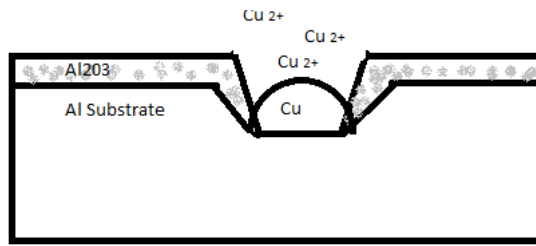
Gambar 3. Mekanisme pembentukan lapisan di celah
