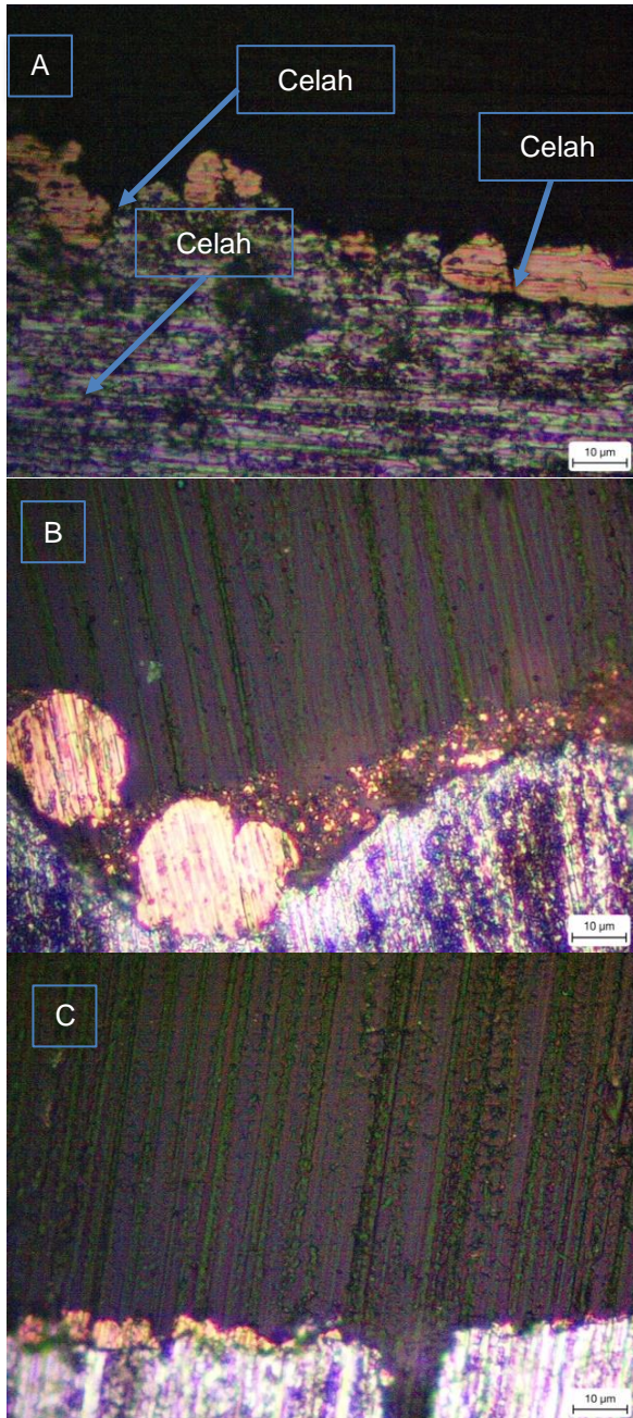
Gambar 2. Hasil electroless plating tembaga pada material aluminium hasil anodisasi selama (A) 13 (B) 26 dan (C) 39 menit terlihat ada celah yang masih terbentuk
