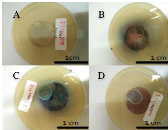
Gambar 5. Penampakan visual hasil Kirby Test dari sampel A) tanpa tembaga B) 13 menit C) 26 menit dan D) 39 menit
