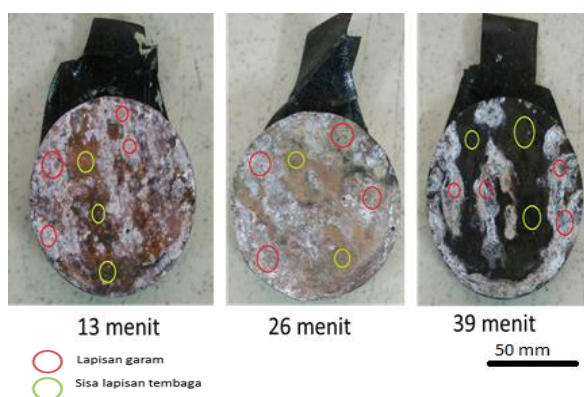
Gambar 7. Penampakan visual hasil uji sembur garam
