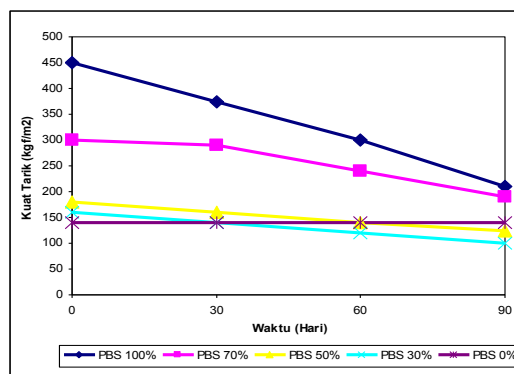
Gambar 4. Perubahan nilai kuat tarik pengujian sifat urai hayati metode soil burial
