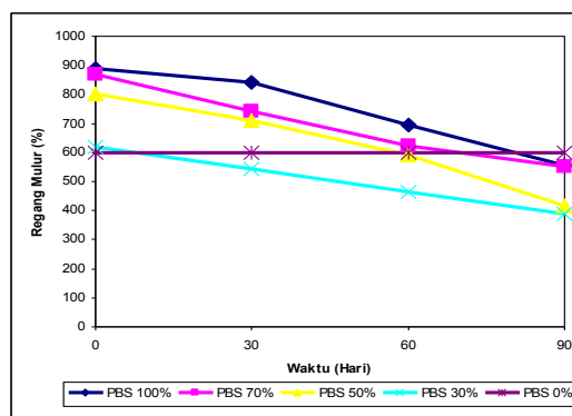
Gambar 5. Perubahan nilai regang mulur pengujian sifat urai hayati metode soil burial
