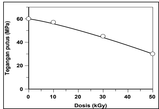
Gambar 2. Hubungan tegangan putus film agar-agar terhadap dosis iradiasi
