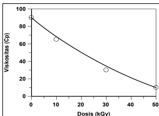
Gambar 1. Hubungan dosis iradiasi terhadap viskositas larutan agar-agar
