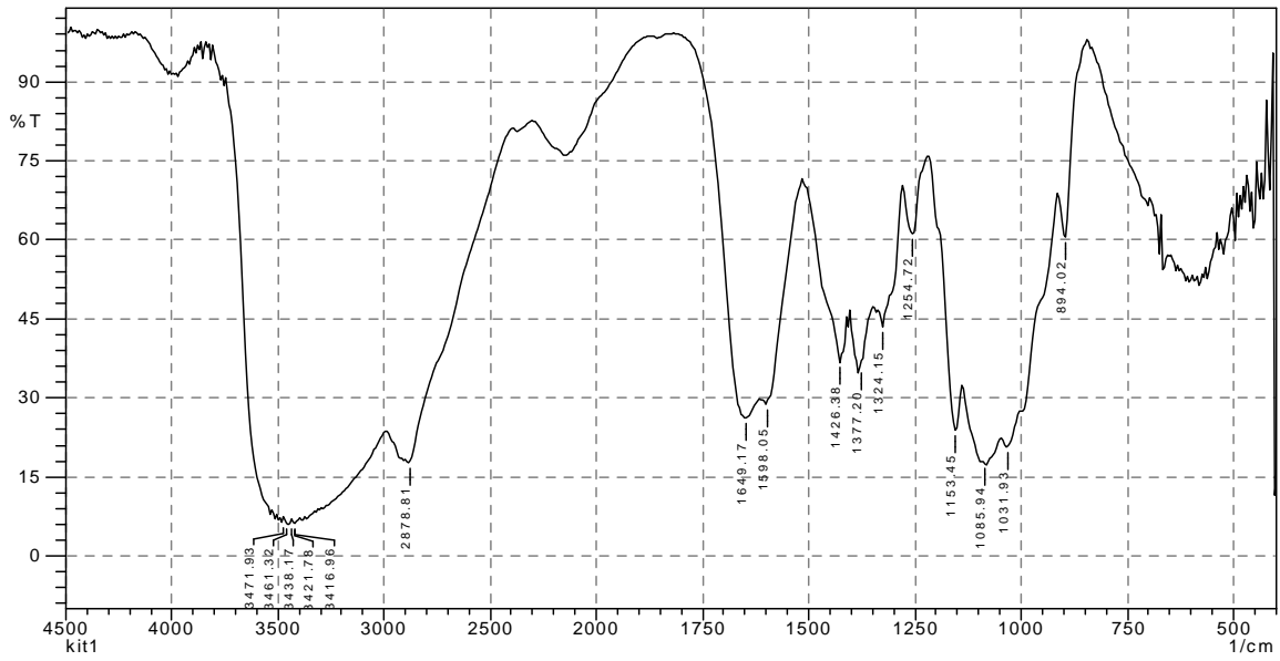
Gambar 3. Kurva FTIR Kitosan
