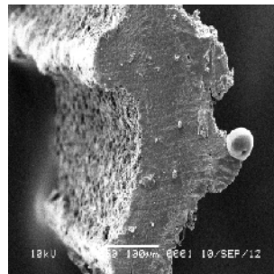
Penampang melintang
