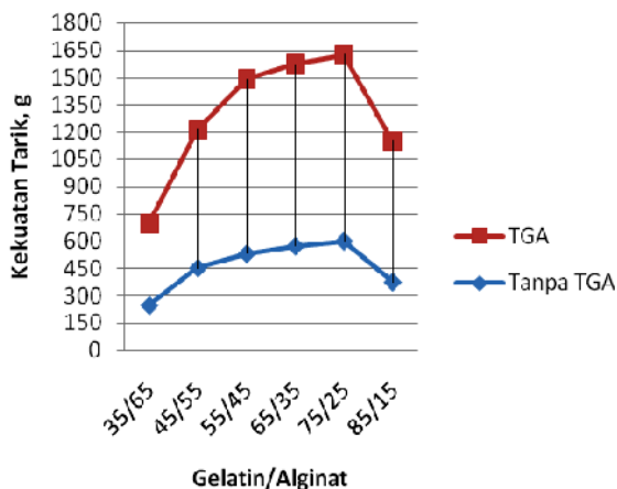
Gambar 4. Hasil Uji Kekuatan tarik Benang Gelatin/Alginate
