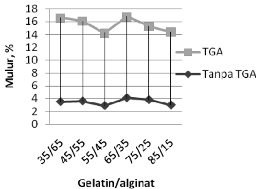
Gambar 7. Hasil Uji Mulur Benang Gelatin/Alginat
