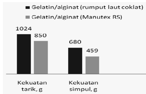
Gambar 6. Hasil Uji Kekuatan Tarik dan Simpul Benang Gelatin/Alginate pada Penggunaan Alginate Hasil ekstraksi dan Alginate Komersil (Manutex RS)
