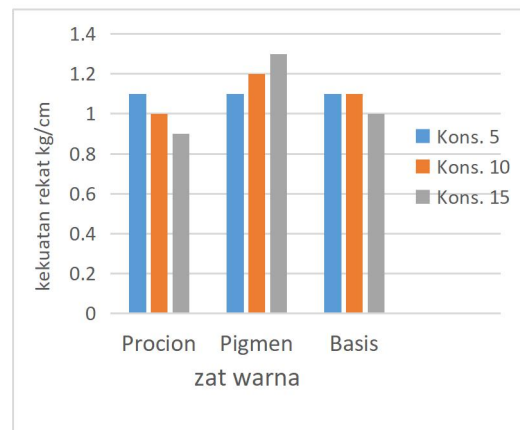
Gambar 4. Histogram Kekuatan Rekat
