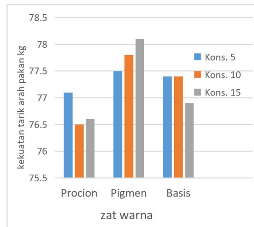
Gambar 6. Histogram Kekuatan tarik arah pakan
